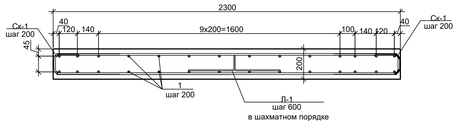
1-1 (Армирование)
