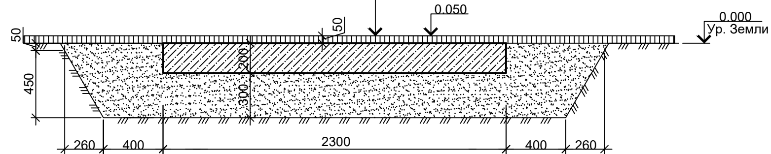
1-1 (Армирование)
