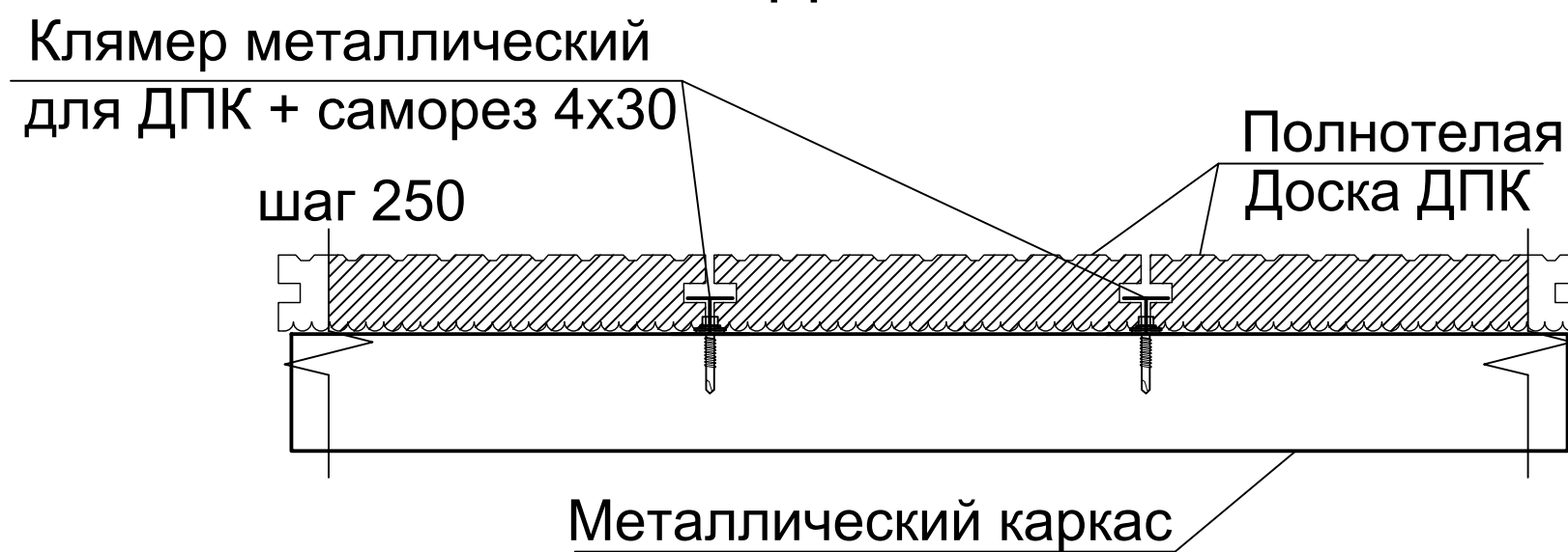
Схема устройства покрытия из террасной доски
