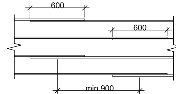
Схема стыковки стержневой арматуры по длине для арматуры Ø12 (соединение арматуры без сварки)
