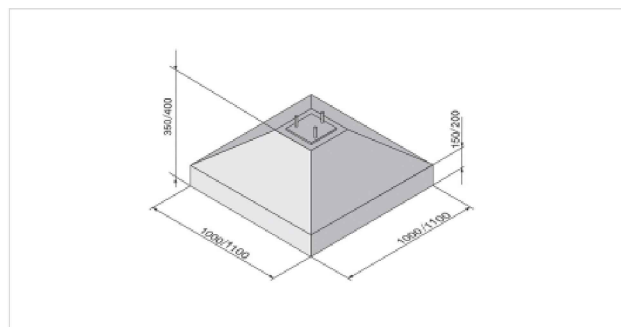
Бетонный блок для флажштоков высотой от 9 до 13 метров (размеры)
