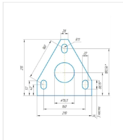
Фланец опоры ø76 3 отверстия М20х160 Лист з/к В ГОСТ14637
