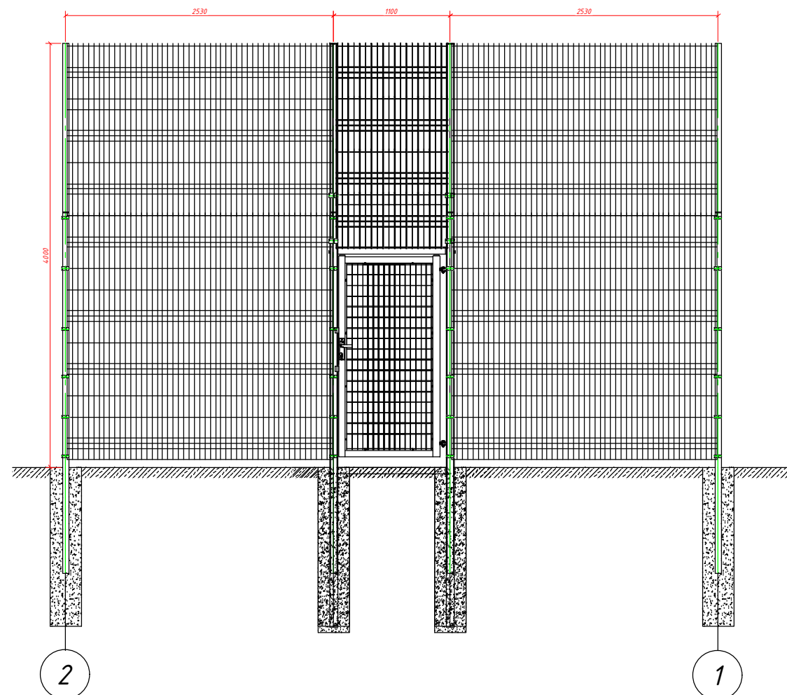
Спортивное ограждение Н=4 м (футбольное поле) стандартные секции и калитка
