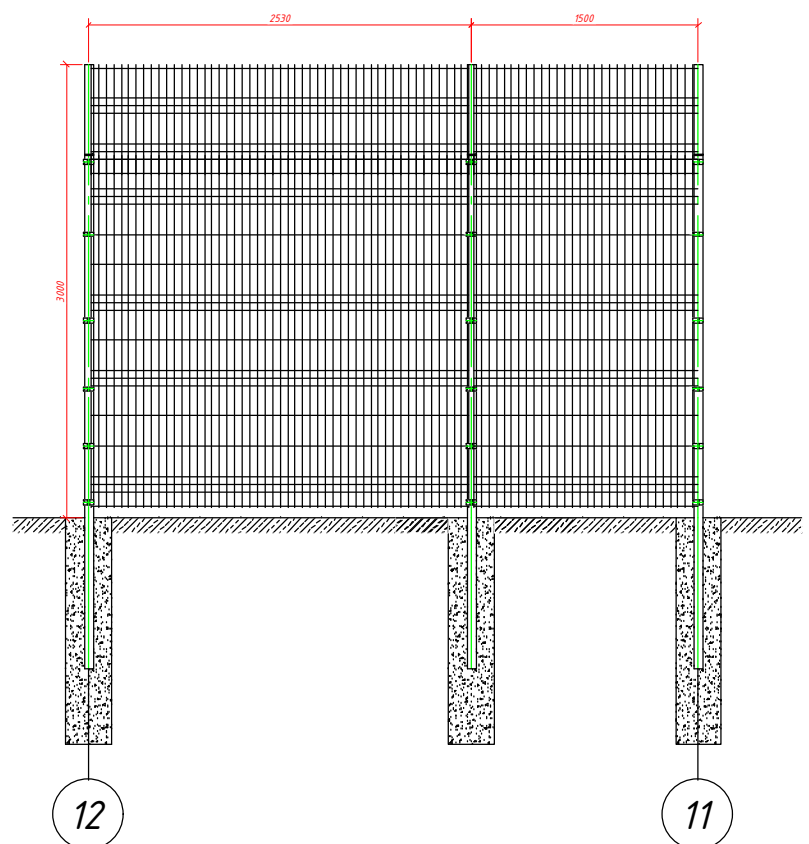
нестандартная секция В=1500мм
