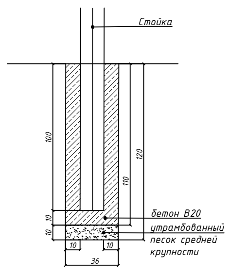
Φ1 Стандартный узел установки игровых элементов М 1:20
