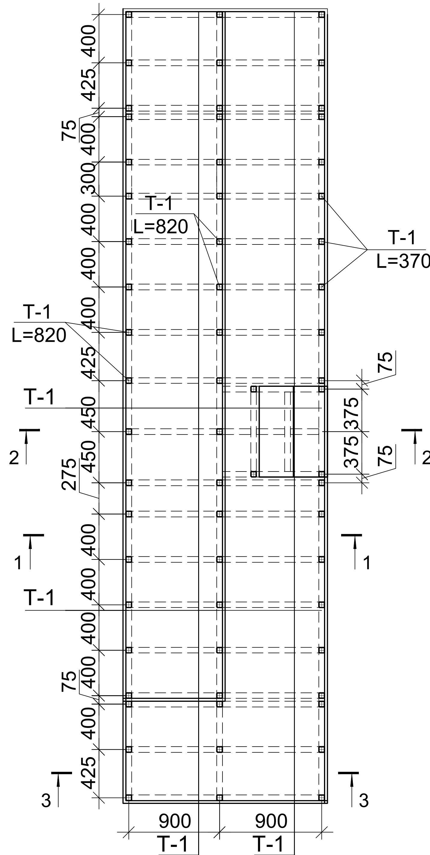
План металлического каркаса амфитеатра
