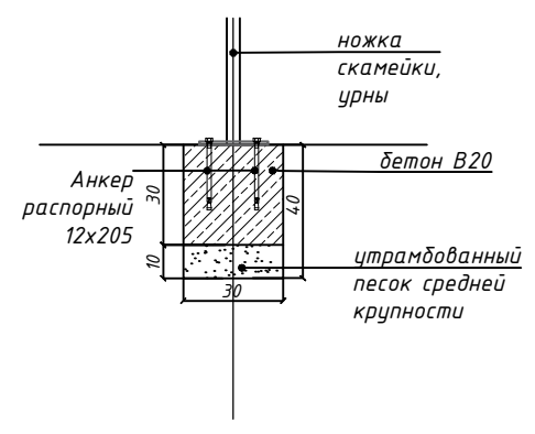
Φ2 Стандартный узел установки скамейки, урны М 1:20
