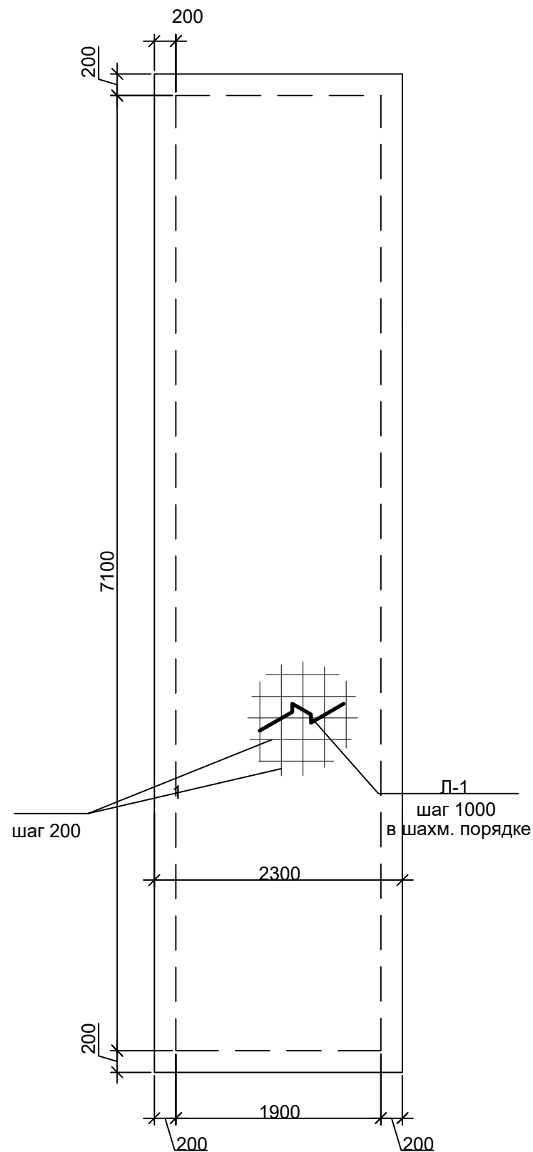
План фундаментной плиты Фп-1 амфитеатра
