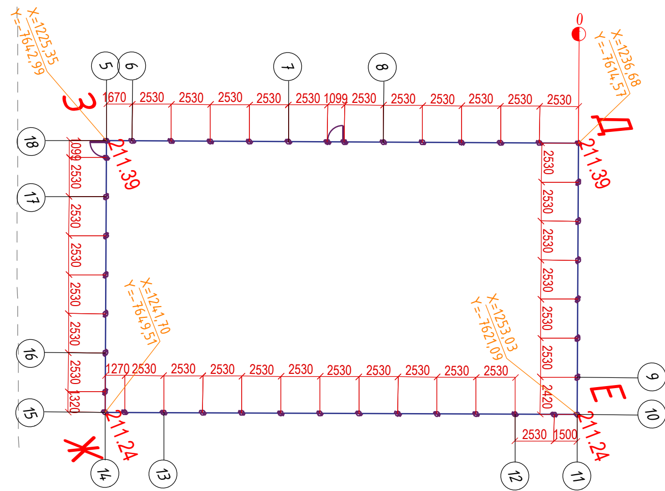
Спортивное ограждение Н=3 м стандартные секции и калитка
