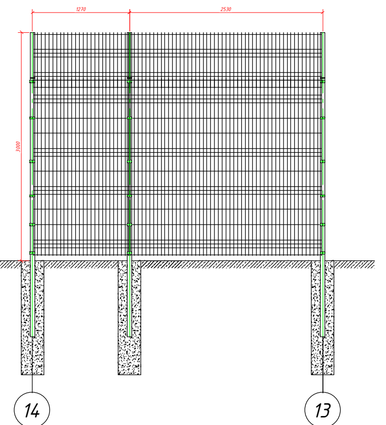
нестандартная секция В=1270мм
