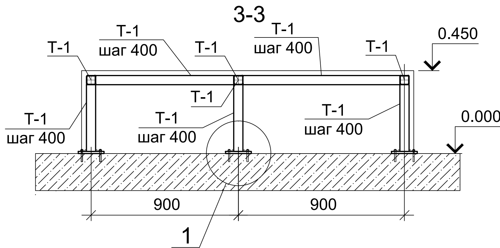
Схема устройства покрытия из террасной доски
