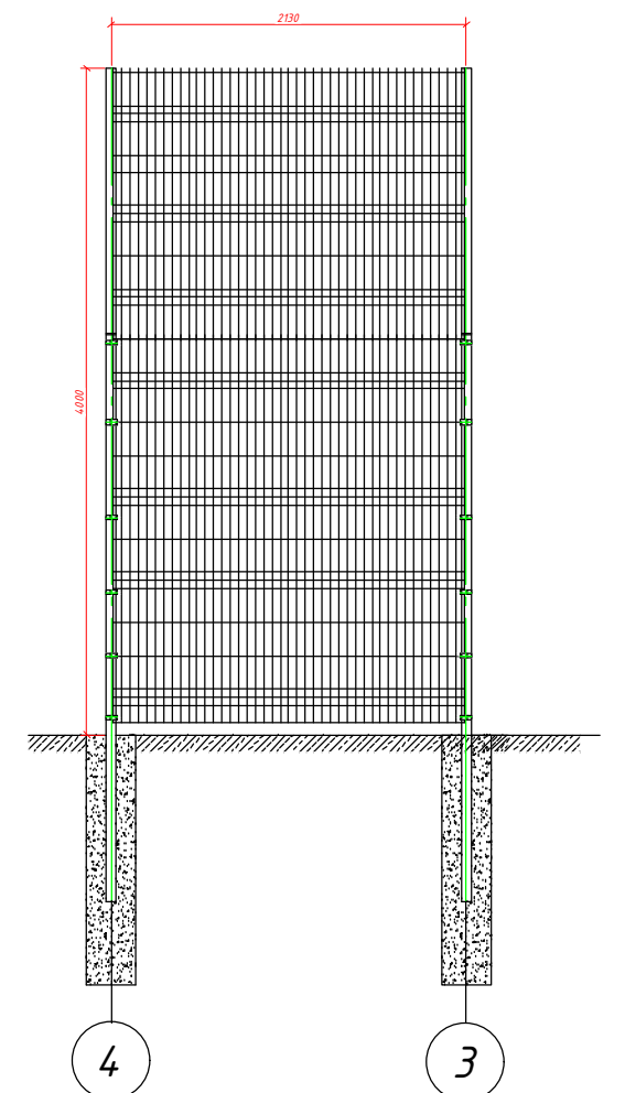
нестандартная секция В=2130
